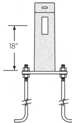
MBQ Elevation
